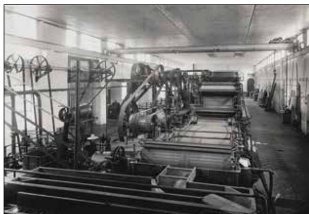
1936 Langsieb-Papiermaschine mit Königswelle und Treibriemen
